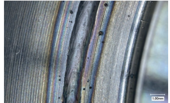
Laserschweißen konventionell conventional laser welding
