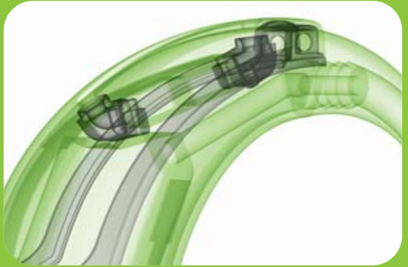
GUMMIFORMTEILE VON KUBO FORM IN EINEM HÖRGERÄT
